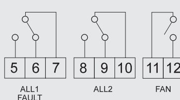
OUTPUTS ALARM RELAYS USCITE RELÈ DI ALLARME
